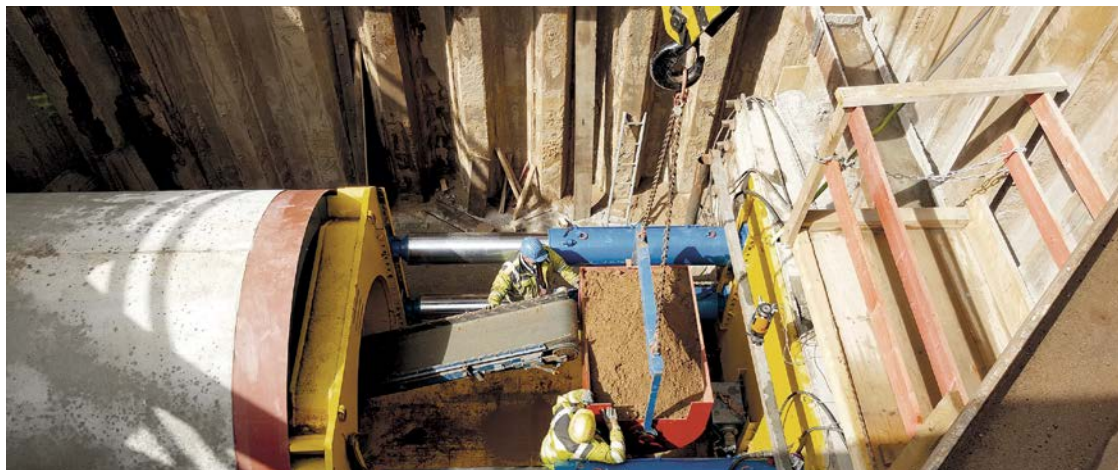
Bodenförderung aus Vortriebsstrecke und Baugrube über Förderband in eine Lore
