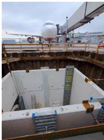
Ortbeton-Ergänzung der Fertigteile im Baufeld
