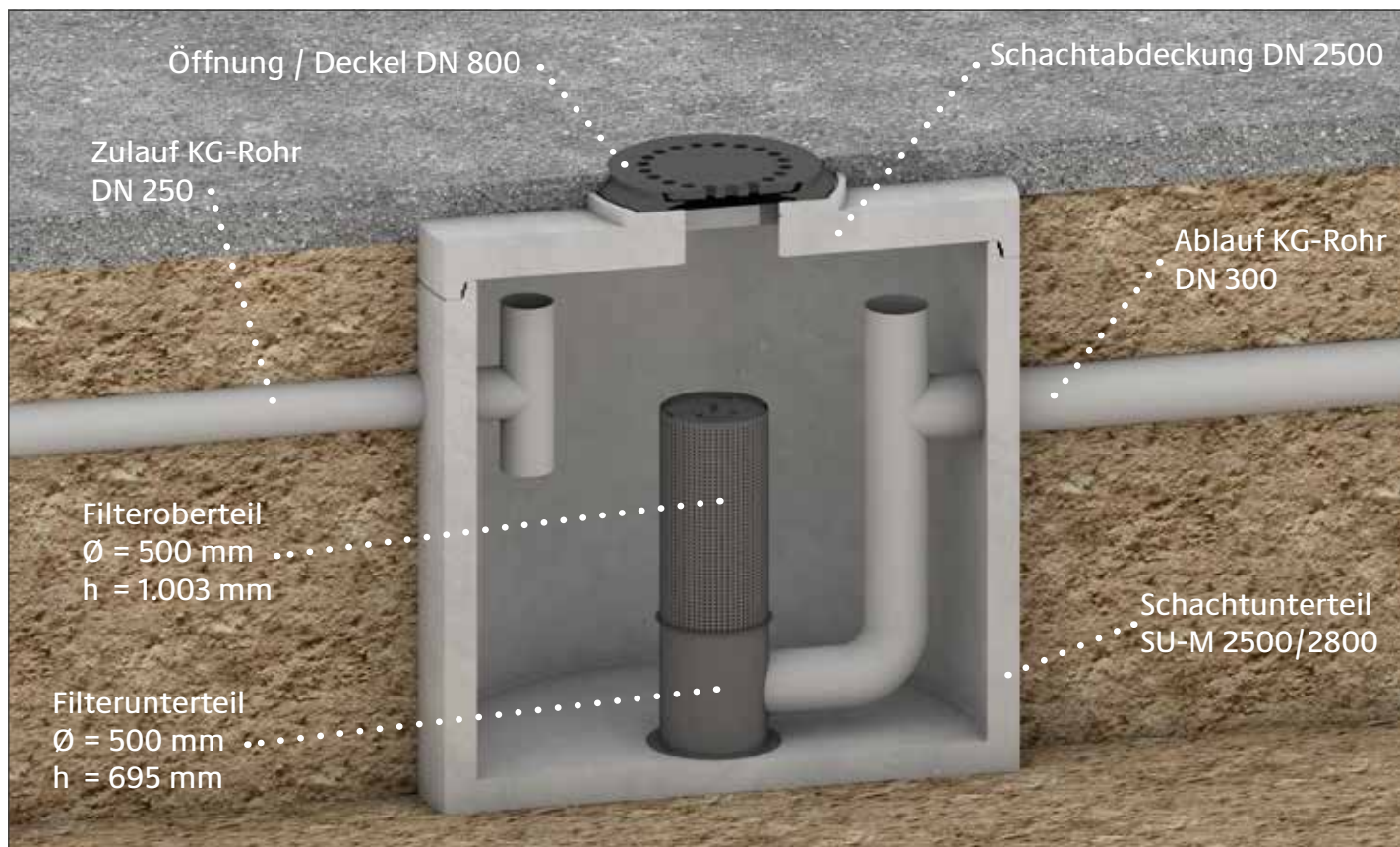
Querschnitt durch den Aufbau des bePlus Systems
