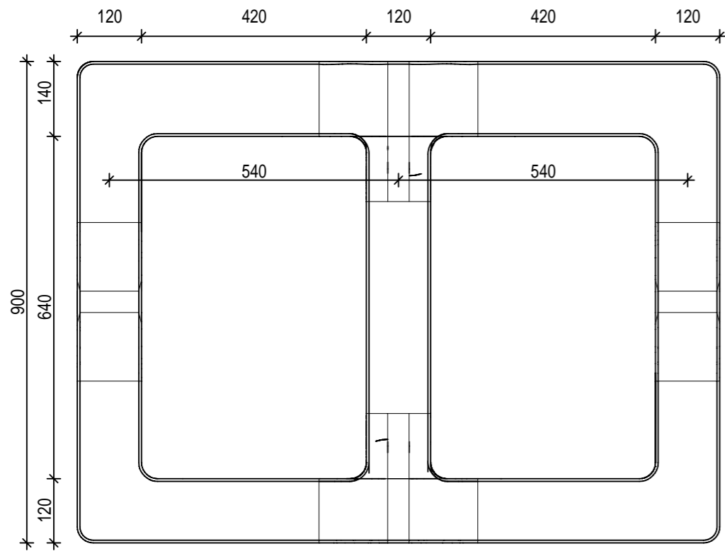
Vorderansicht
